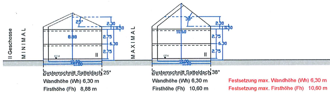
Abbildung: Gebäudesystemschnitte, o.M.
